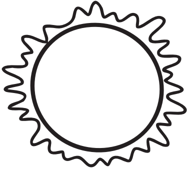
SUN
