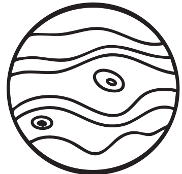
JUPITER
